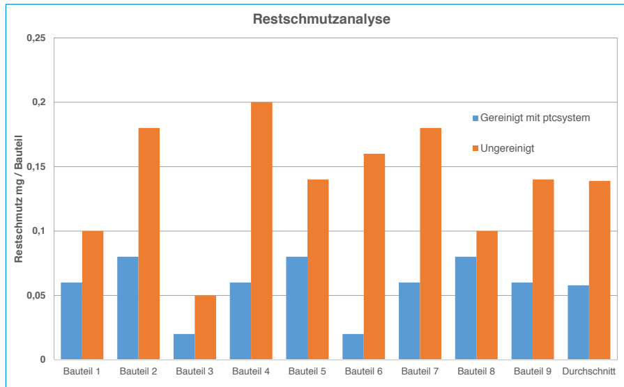
Restschmutzanalyse eines Automobilzulieferers an jeweils neun mit dem ptcsystem ® gereinigten und ungereinigten Hydraulikleitungen.
